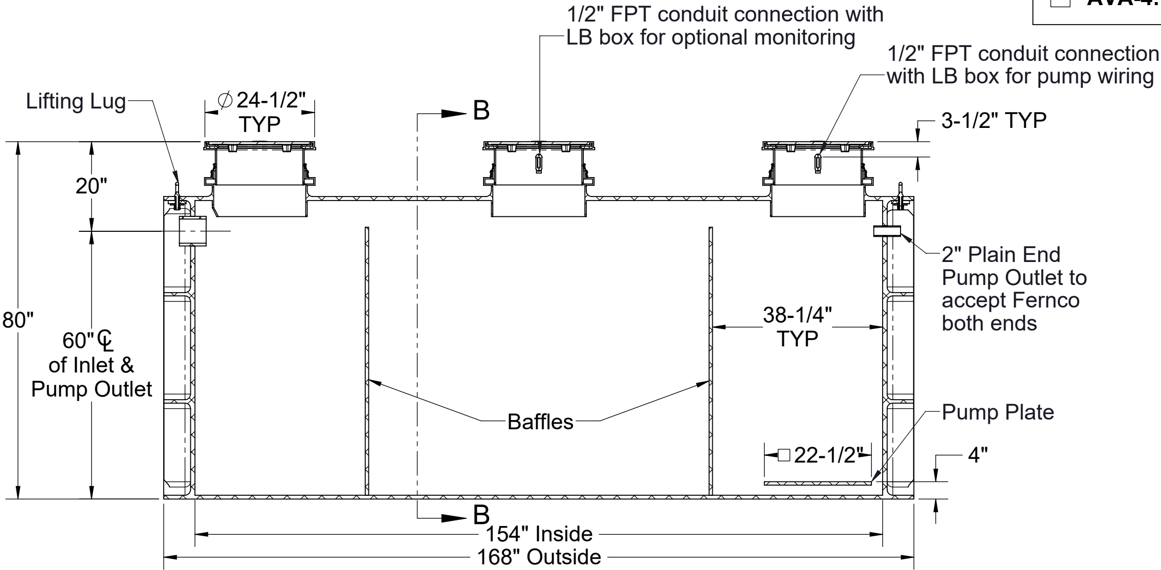
SECTION A-A
