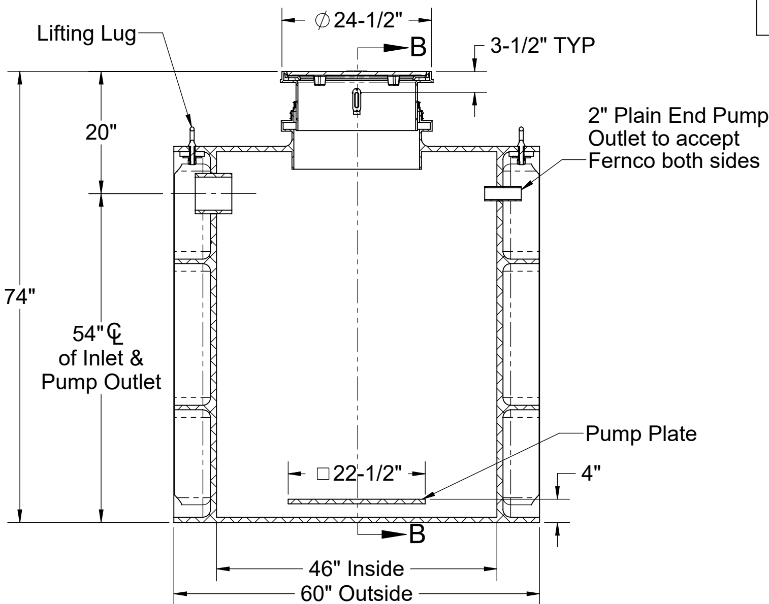
SECTION A-A
