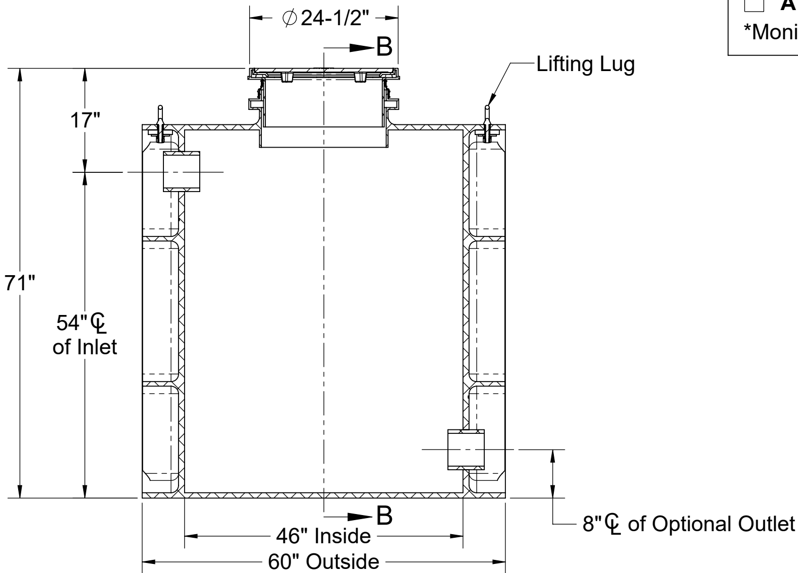
SECTION A-A
