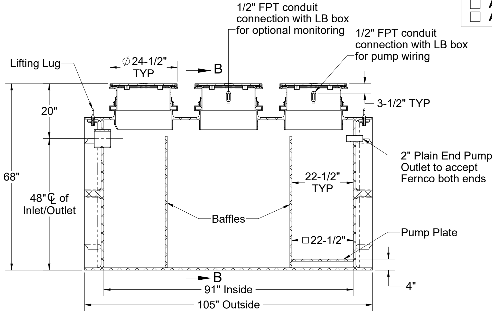
SECTION A-A
