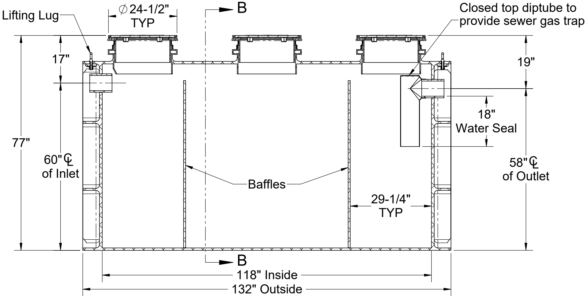
SECTION A-A
