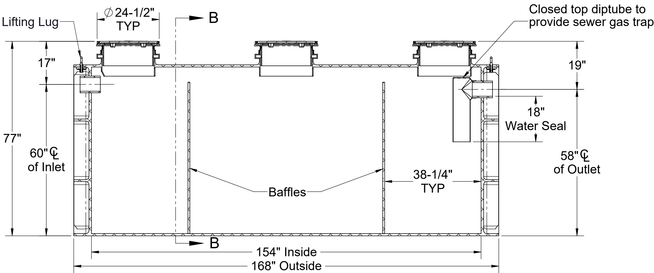
SECTION A-A
