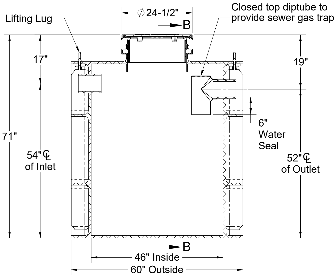
SECTION A-A
