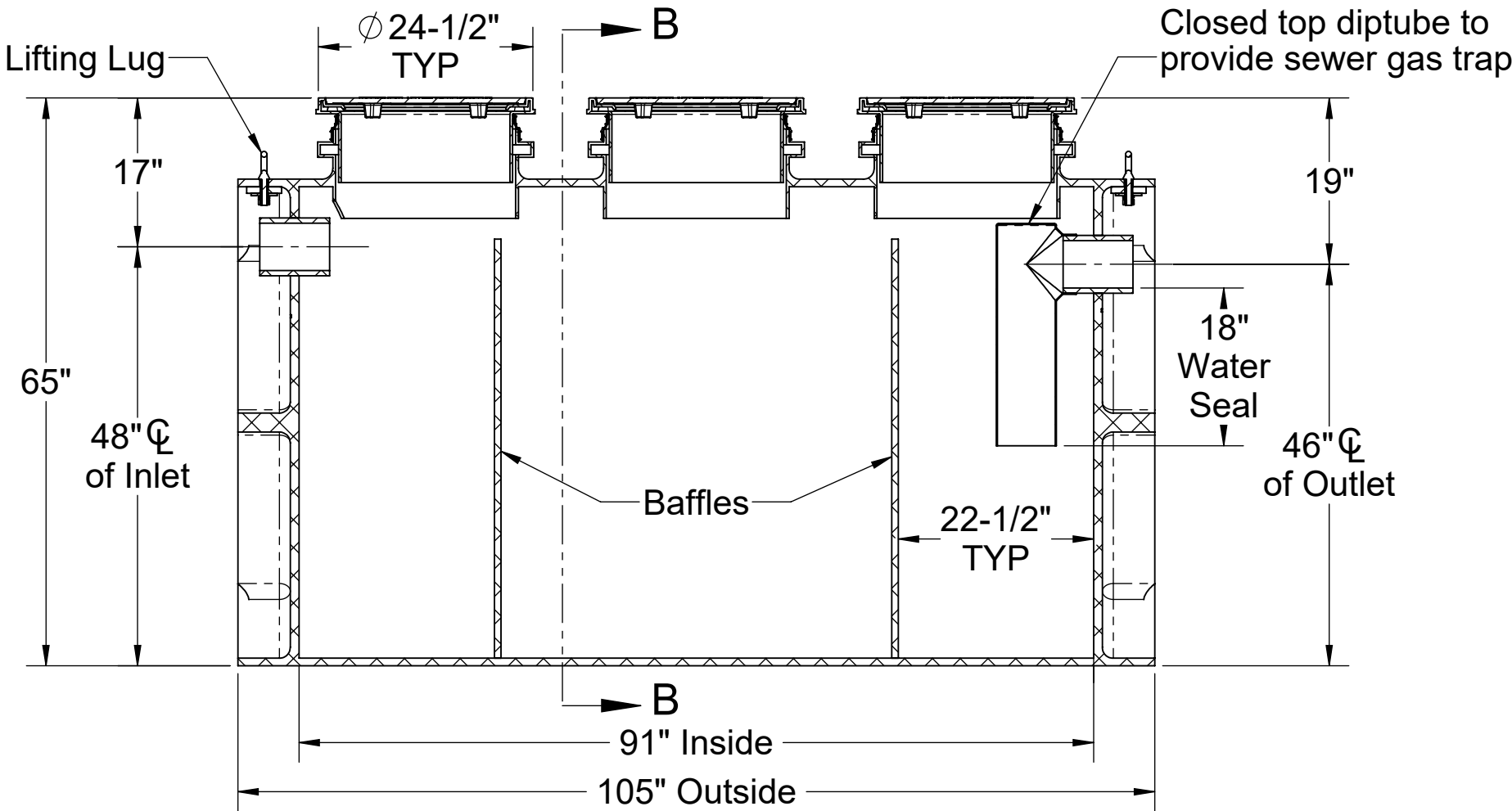
SECTION A-A
