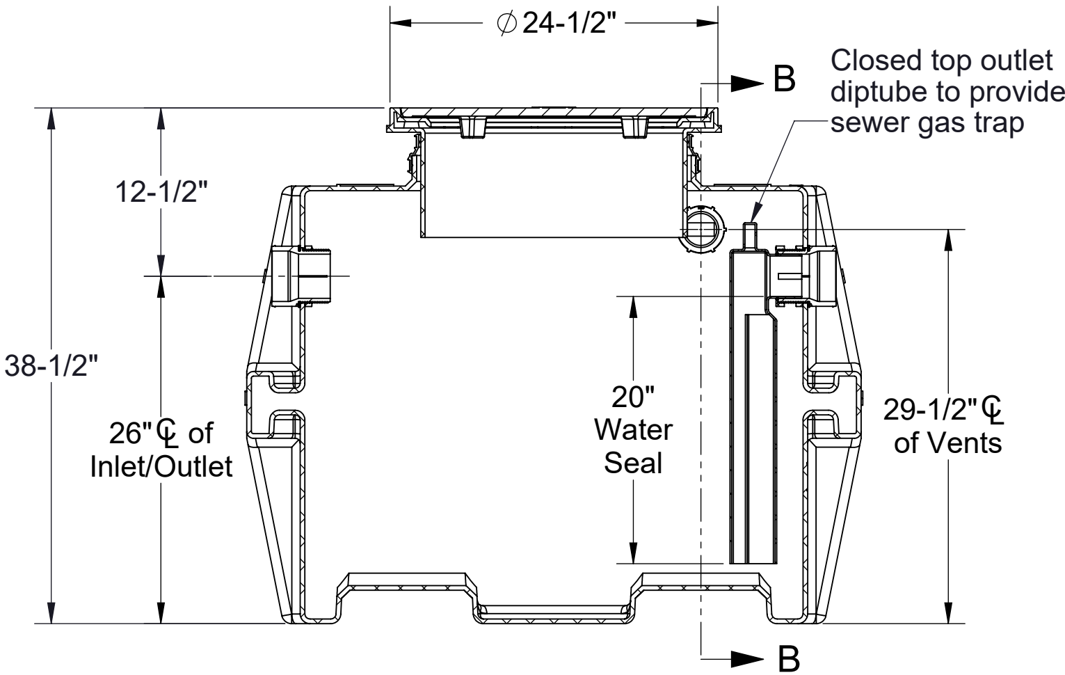
SECTION A-A
