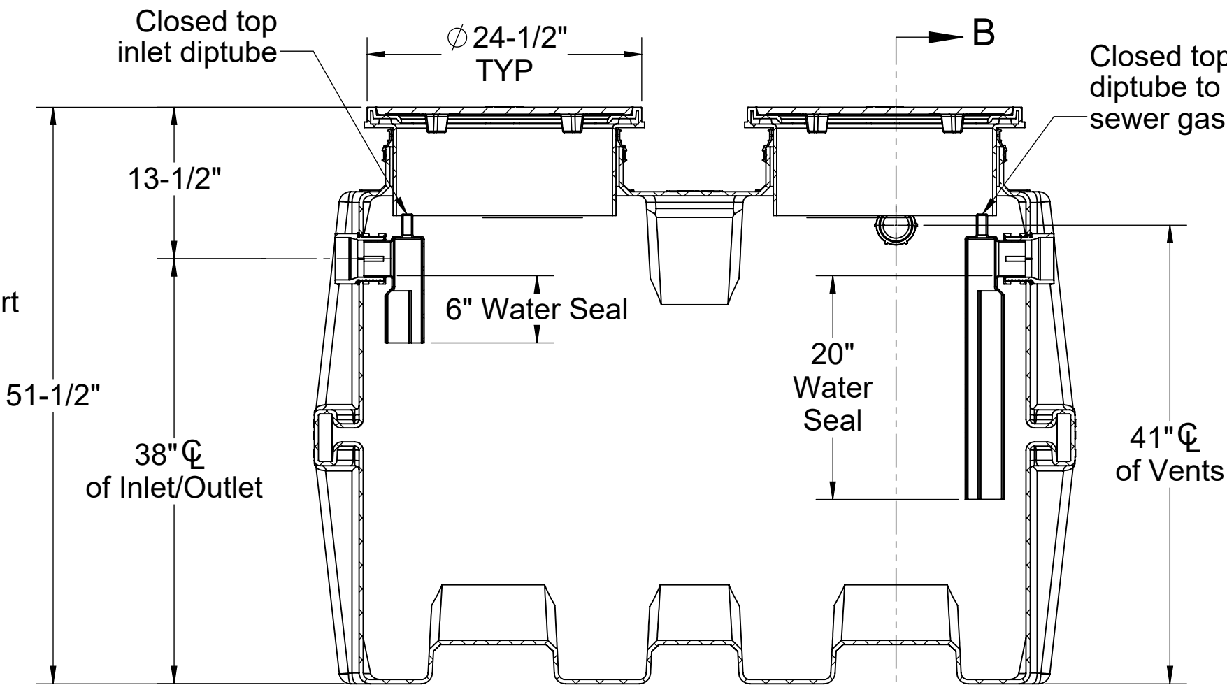
SECTION A-A
