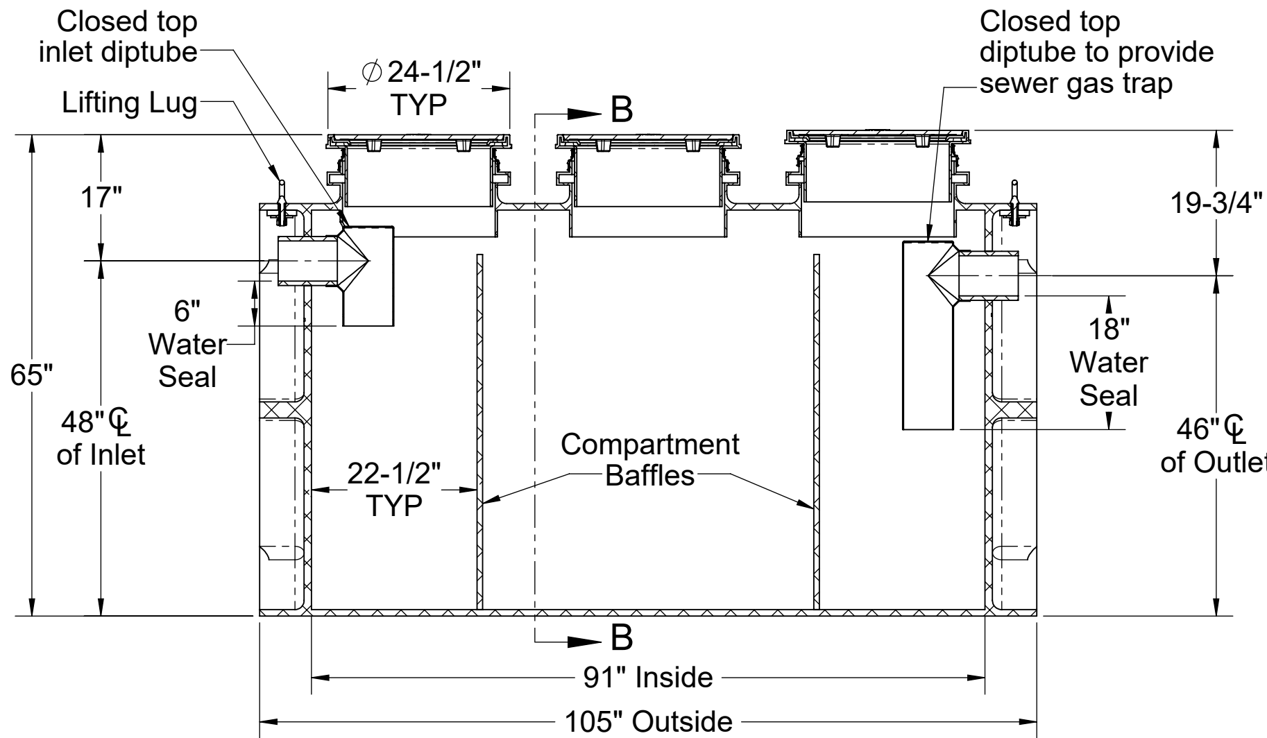
SECTION A-A
