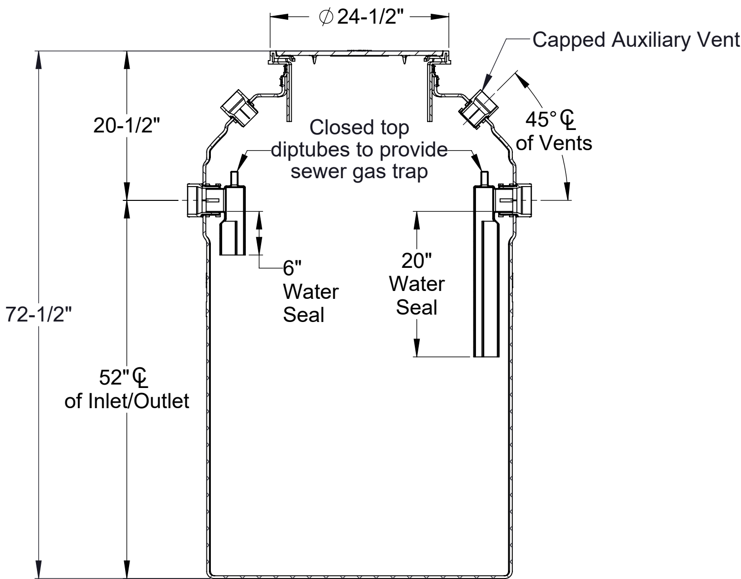
SECTION A-A
