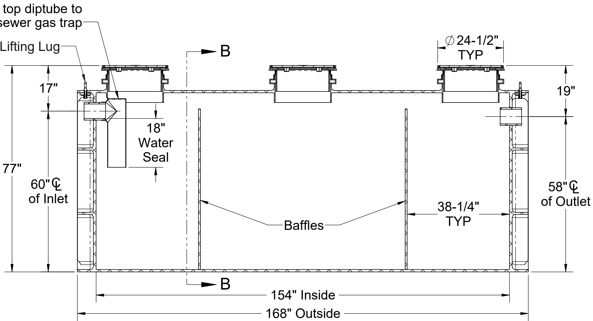
SECTION A-A
