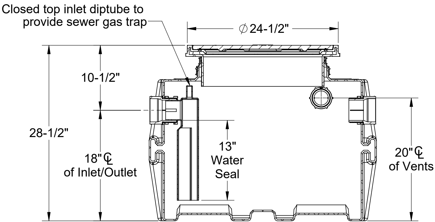
SECTION A-A
