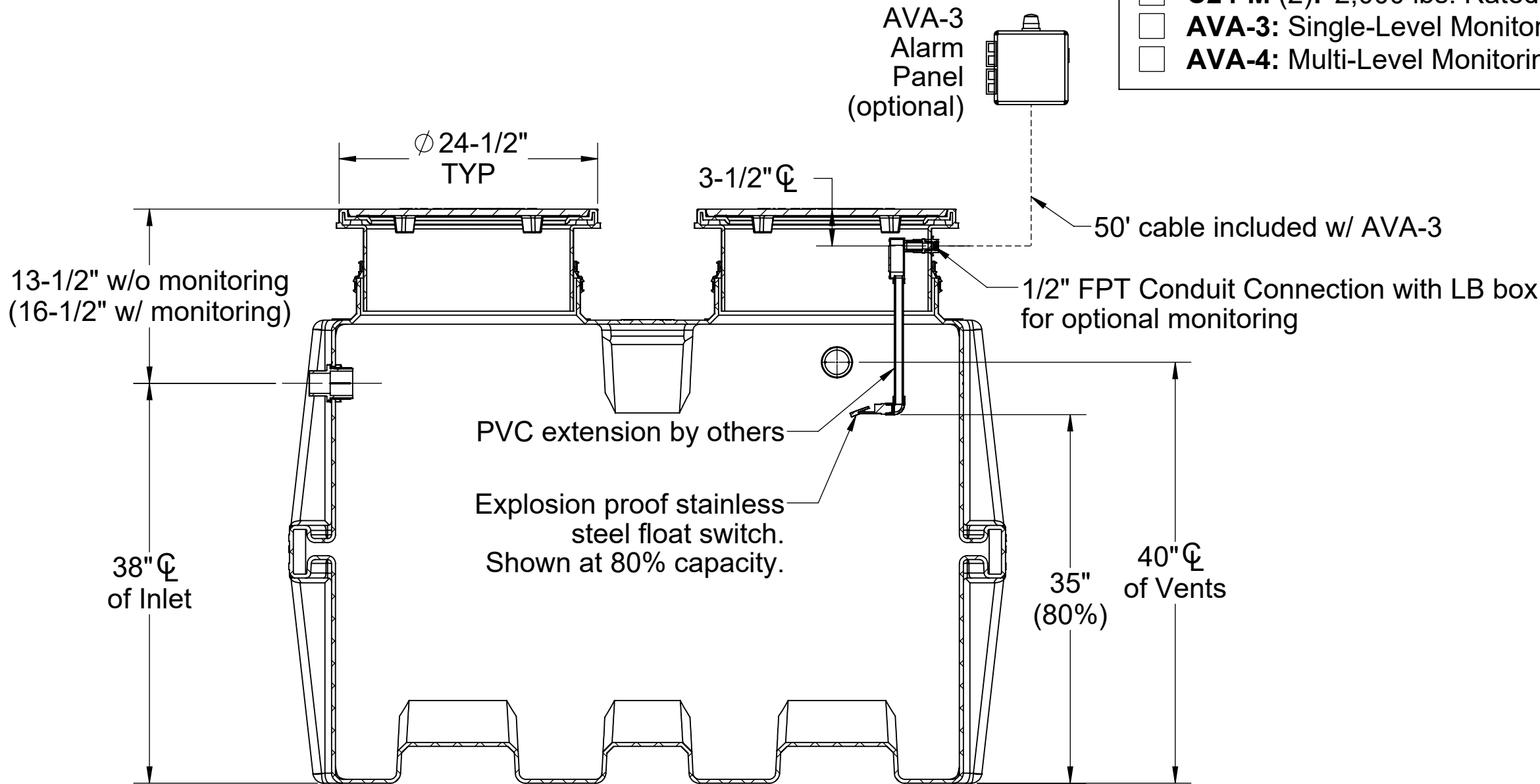
SECTION A-A
