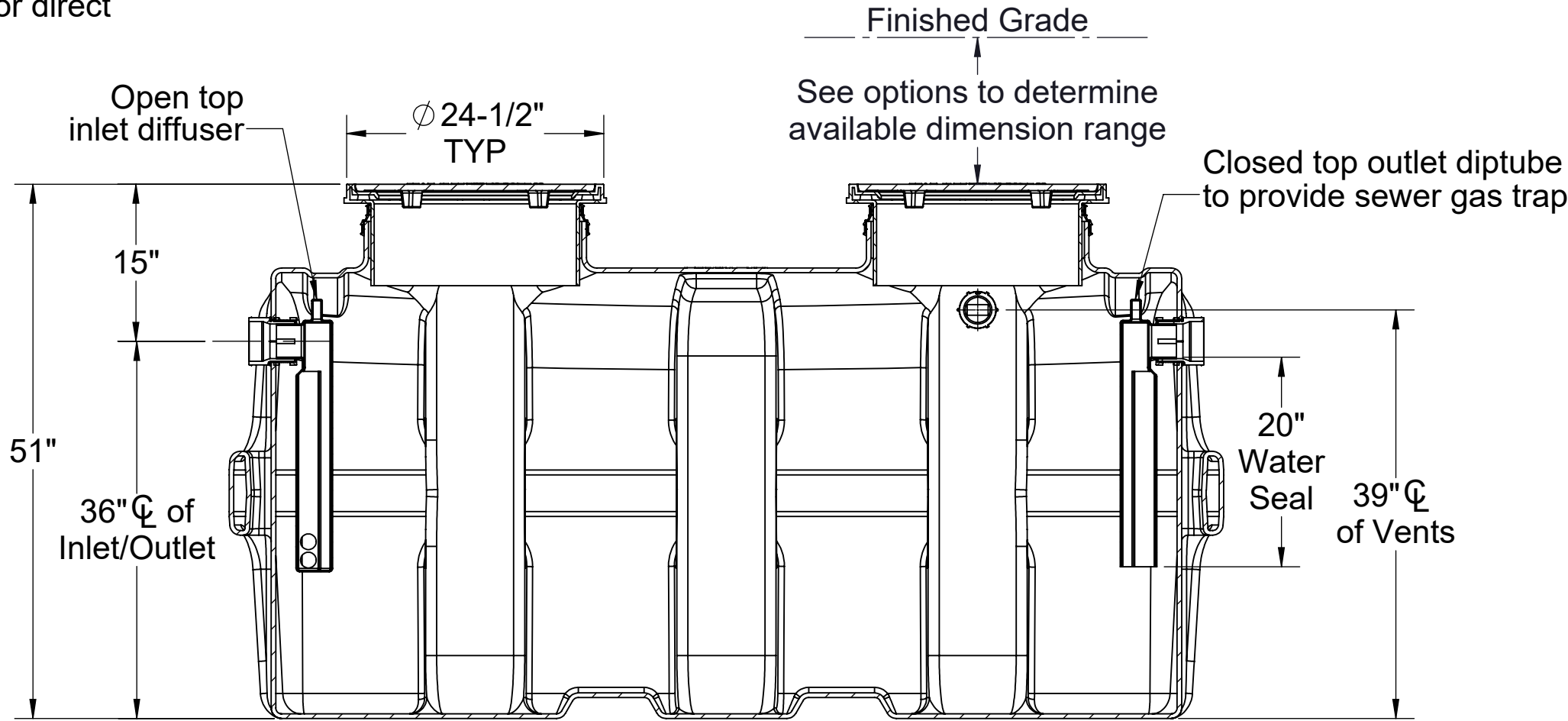
SECTION A-A
