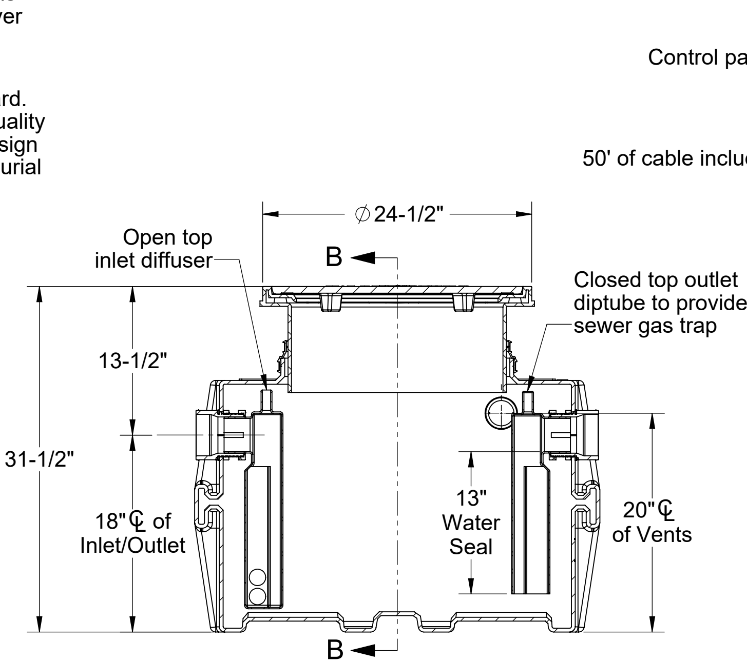
SECTION A-A
