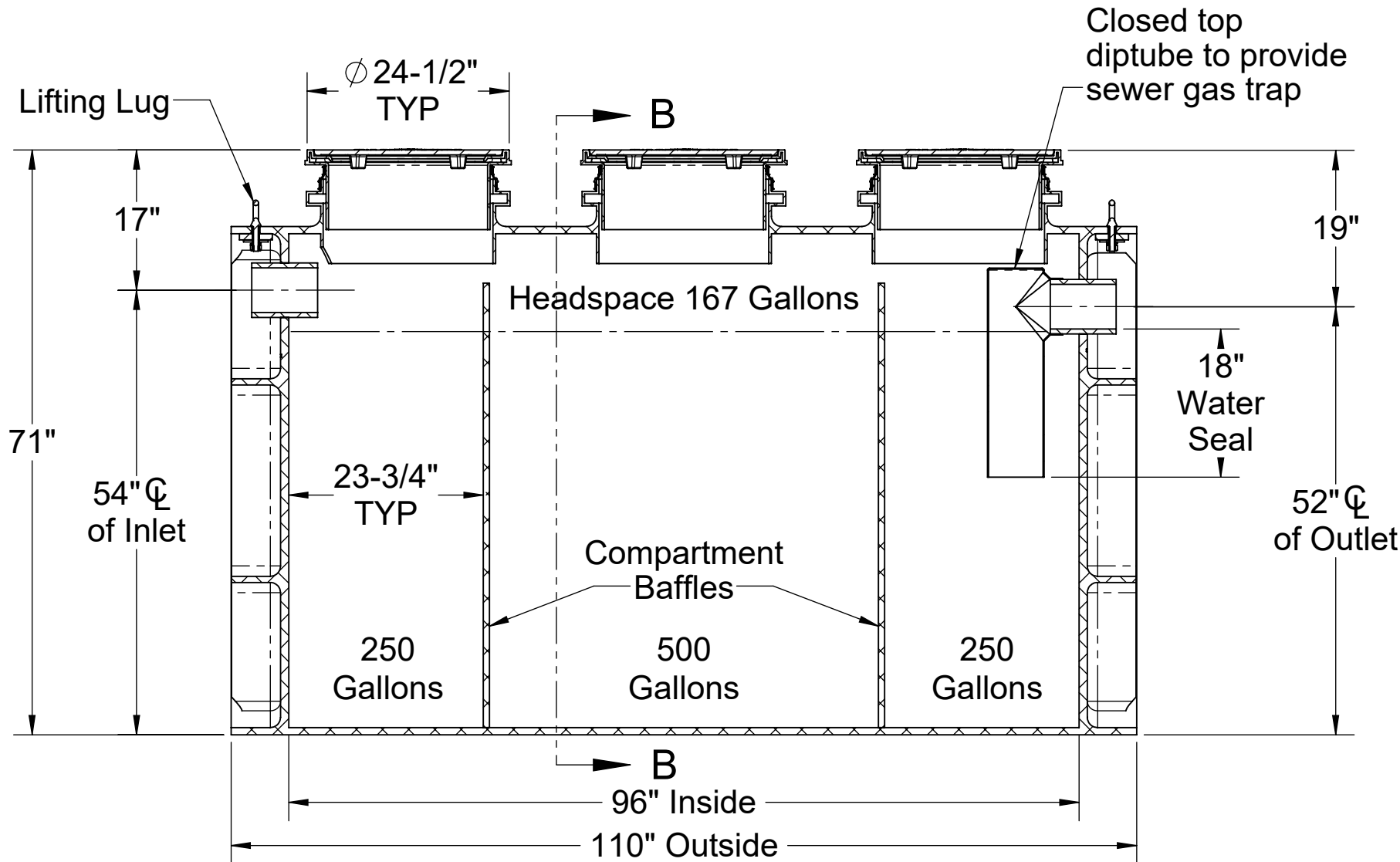
SECTION A-A
