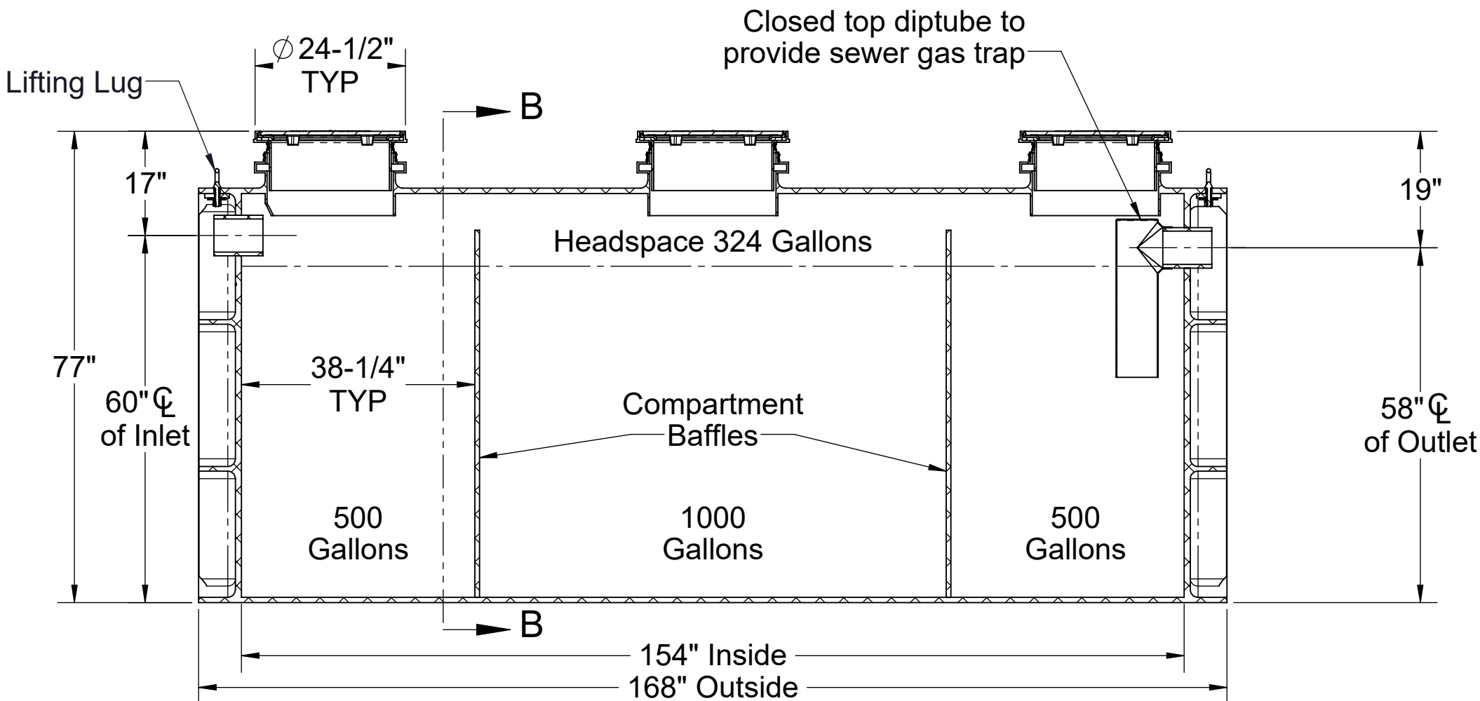
SECTION A-A
