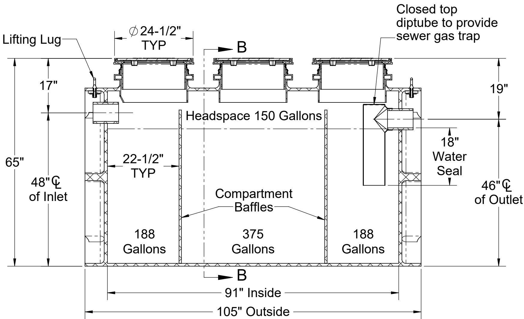
SECTION A-A
