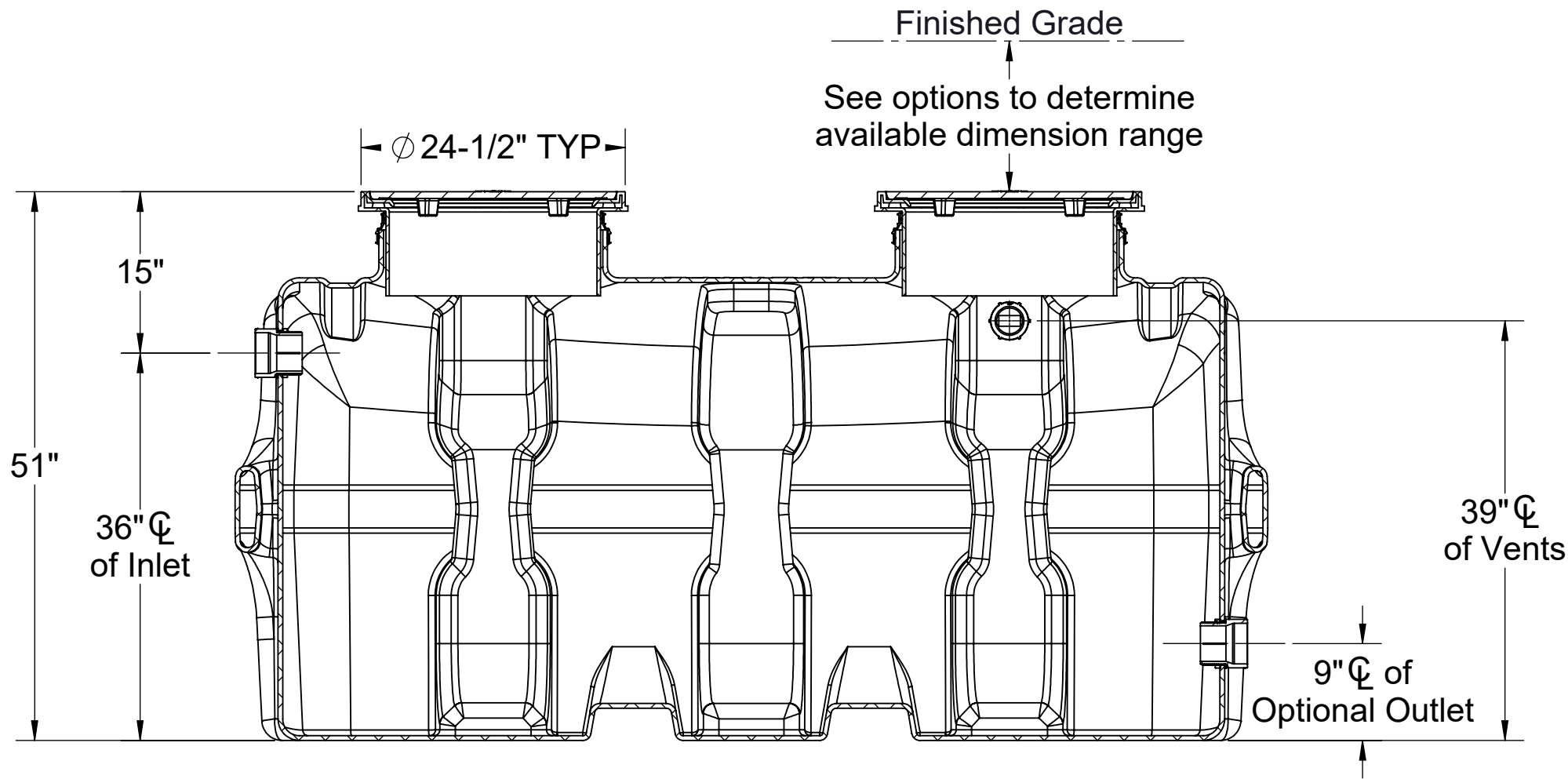
SECTION A-A
