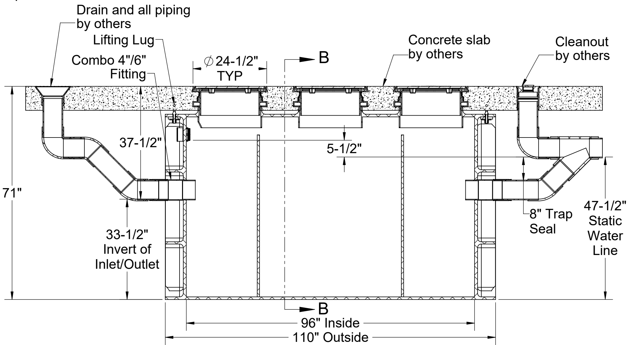
SECTION A-A
