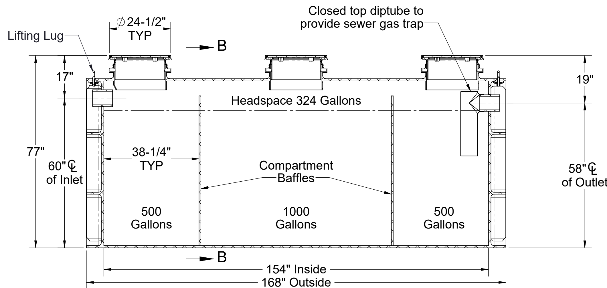
SECTION A-A
