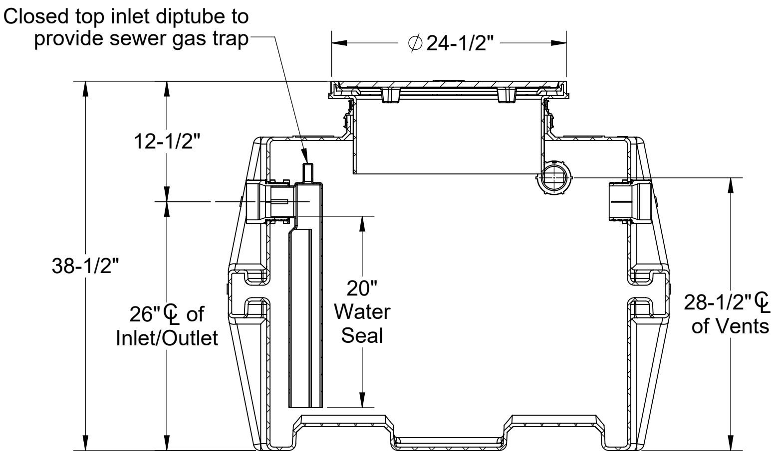
SECTION A-A
