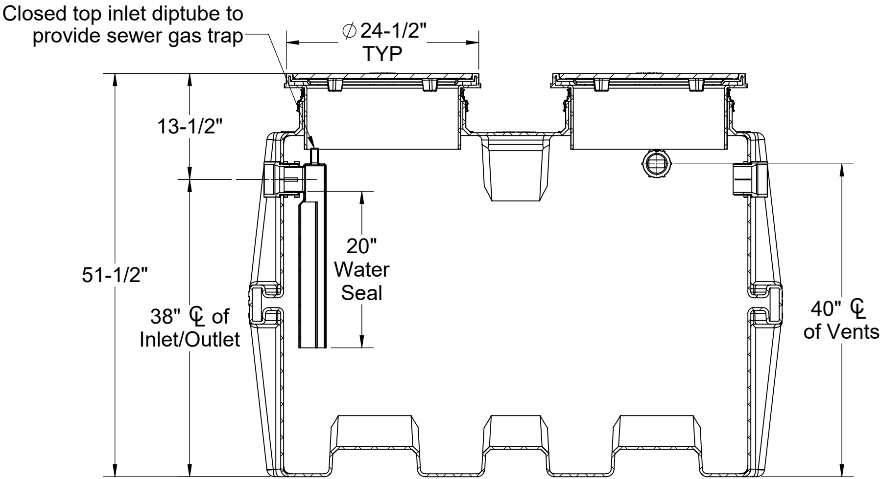
SECTION A-A
