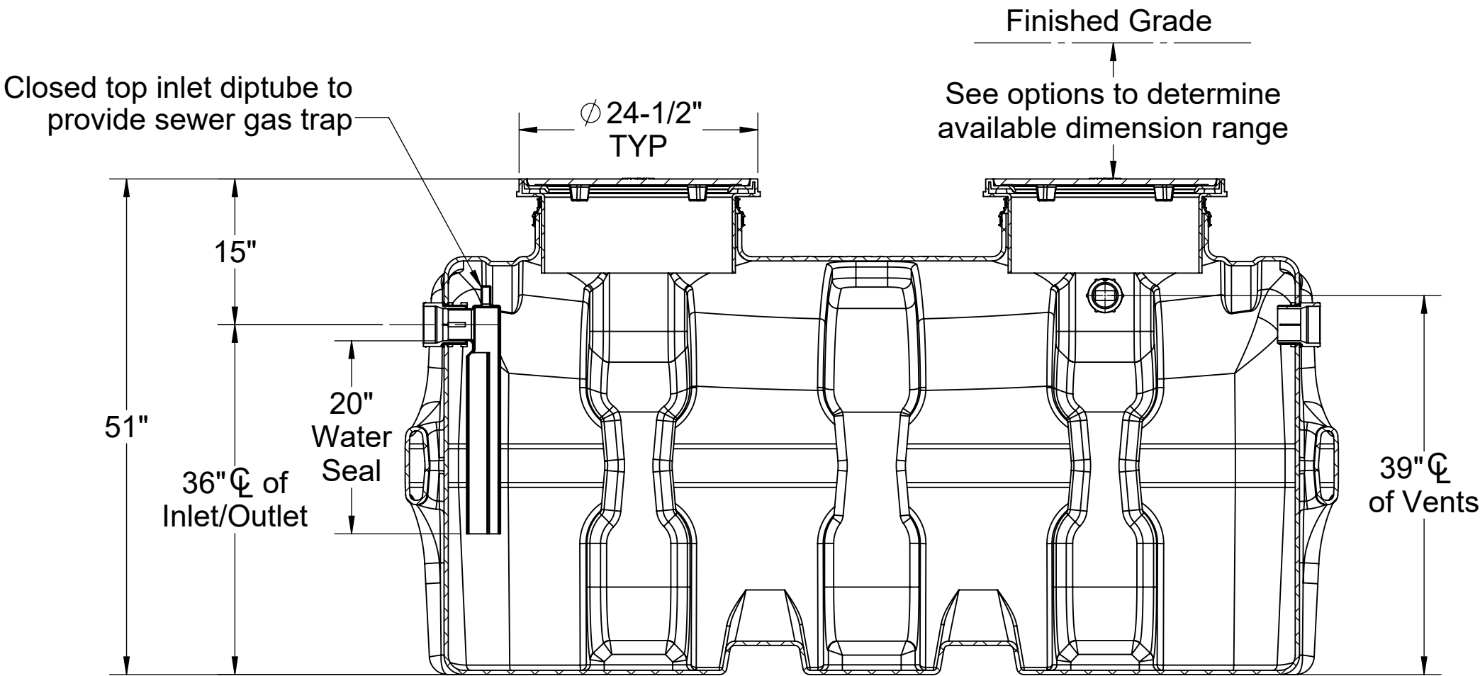
SECTION A-A
